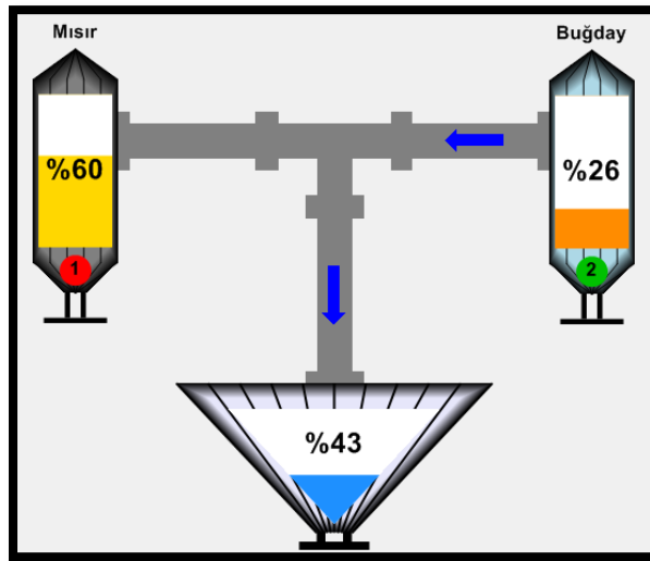
Silo, Karıştırma Tankı ve Boru Bileşenleri
